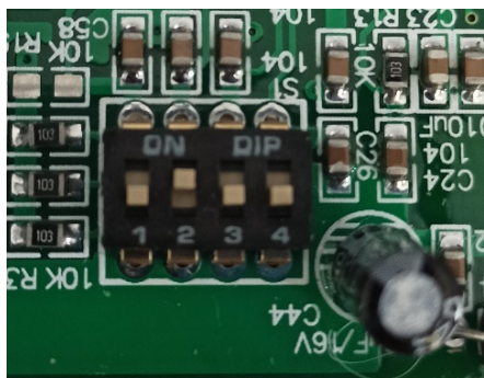
Рис. 9 Колодка переключателей S1 на плате электронной
